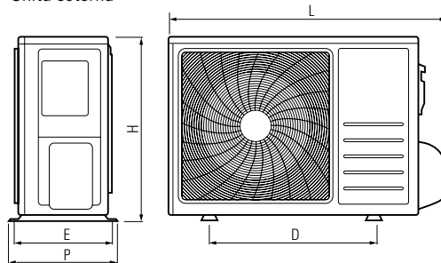
Unità esterna
