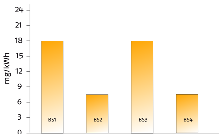
EMISSIONI DI CO (gas G20)
