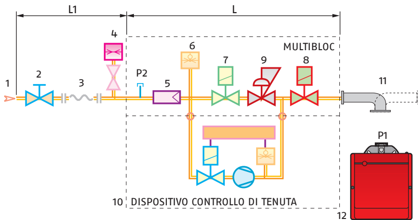
Rampa gas installata sul bruciatore
